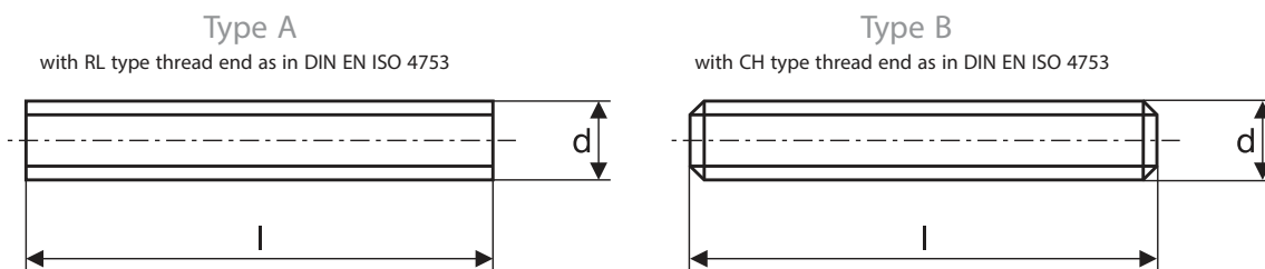
DIN 976-1 Stud bolt dimensions
